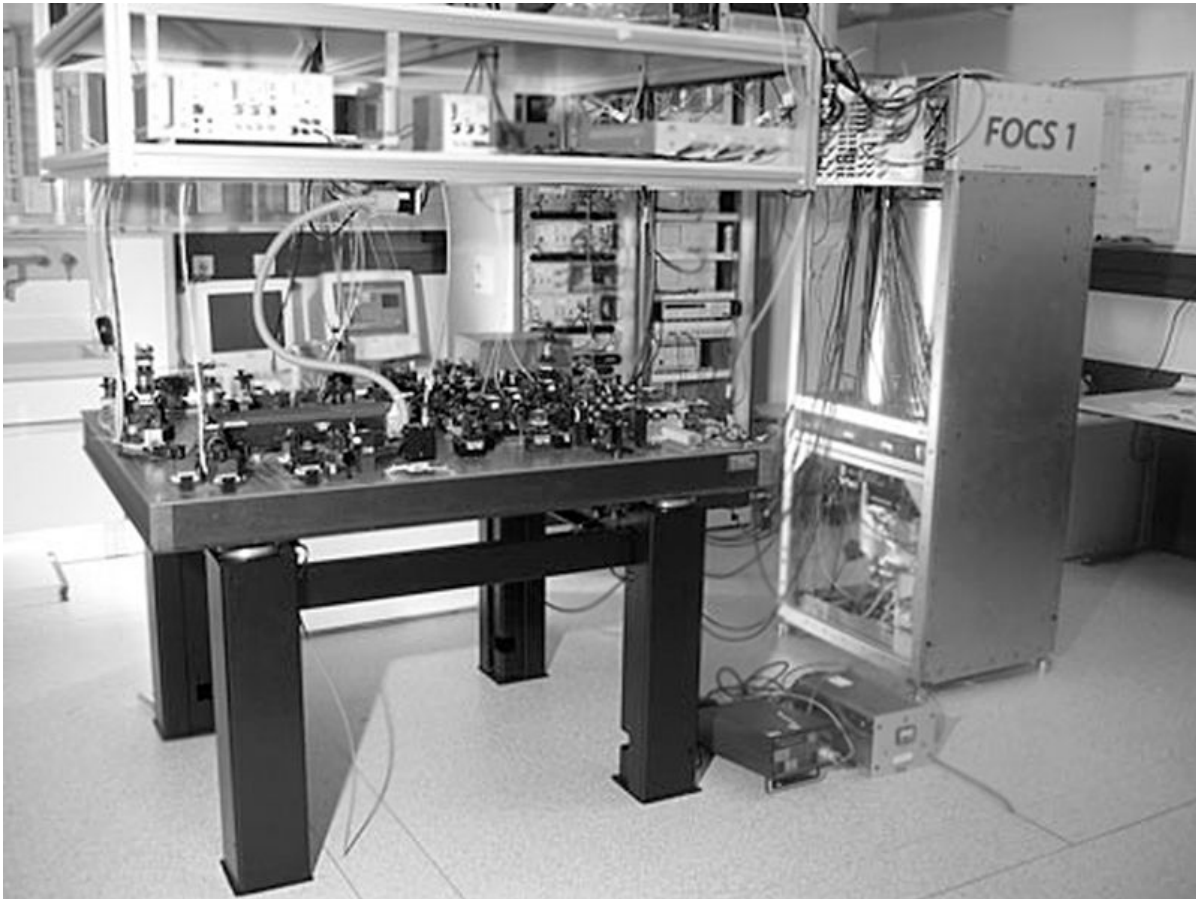
Orologio atomico al cesio costruito nel 2004 per un laboratorio svizzero che opera con un'incertezza di 1 secondo ogni 30 milioni di anni.
